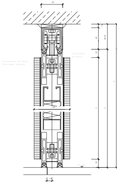
1-Punktschiene
