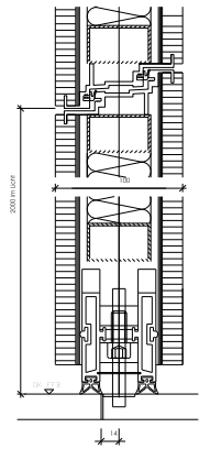
Türenelement
